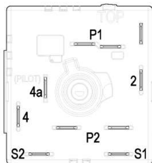
Lage der Flachstecker für die neuen Energieregler
