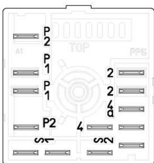
Lage der Flachstecker für die alten Energieregler
